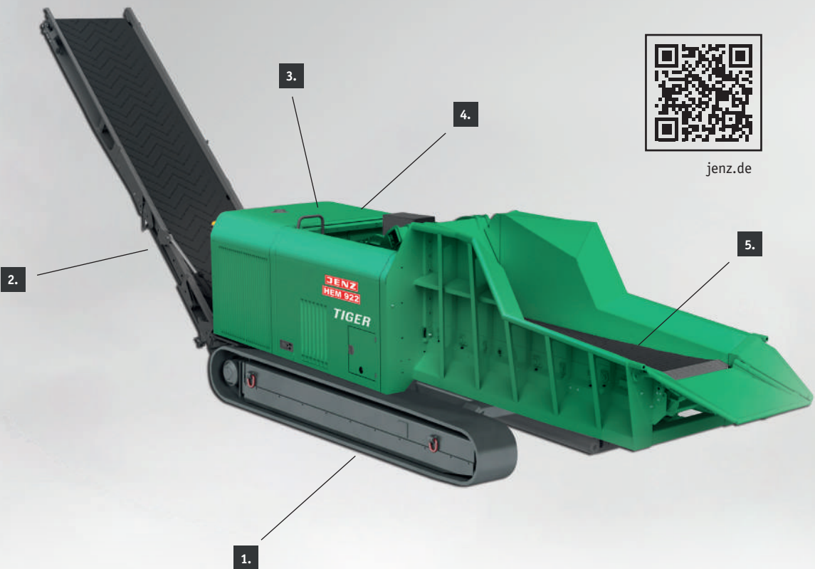
1. Selbständiges Bewegen auf festem, unebenen Boden Self-propelled movement on solid, uneven ground 2. Materialaustrag über Förderband Material outfeed using Conveyor belt
